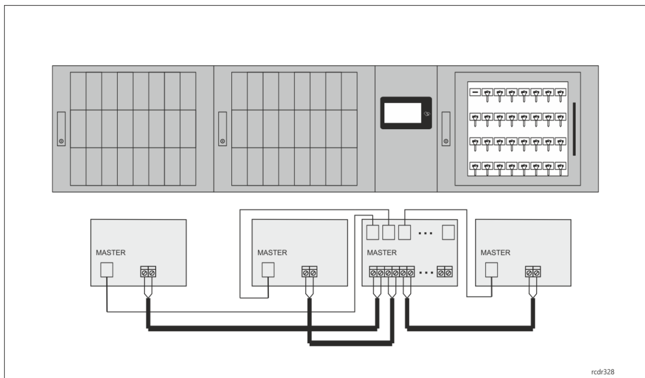
Rys. 10 Podłączenie dodatkowych szaf (RKD24CT-EXT, RKD32EXT) do depozytora (RKD24CT)
